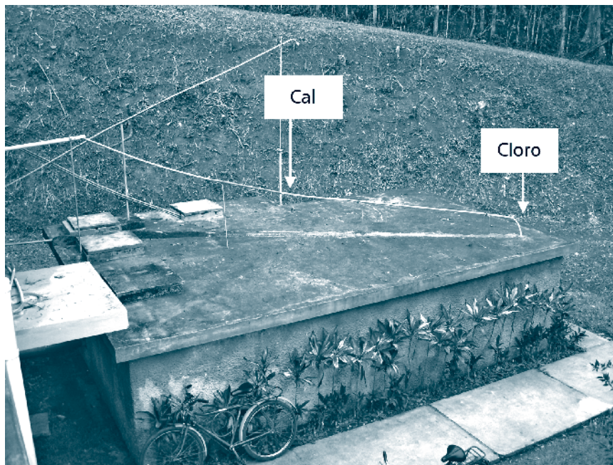
Figura 2.32 – Aplicação correta de produtos químicos no tanque de contato: "cloro" – gás na entrada e "cal" na saída
