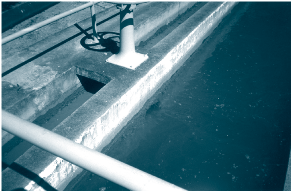
Figura 2.27 – Dispositivo inadequado de entrada de água floclada no decantador, provocando quebra de flocos
