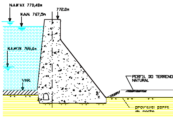
CORTE TRANSVERSAL TÍPICO ESC 1:500
