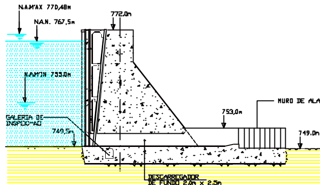
DESCARREGADOR DE FUNDO PARA DESVIO CORTE LONGITUDINAL ESC 1:500
