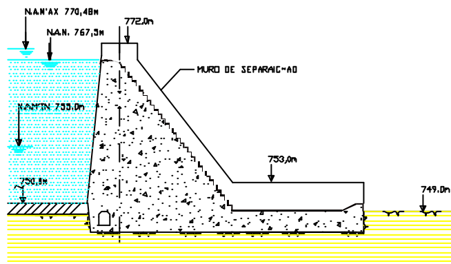
VERTEDOURO CORTE TRANSVERSAL ESC 1:500
