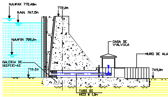
CONTROLE DE VAZÃO PARA JUSANTE CORTE LONGITUDINAL ESC 1:500
