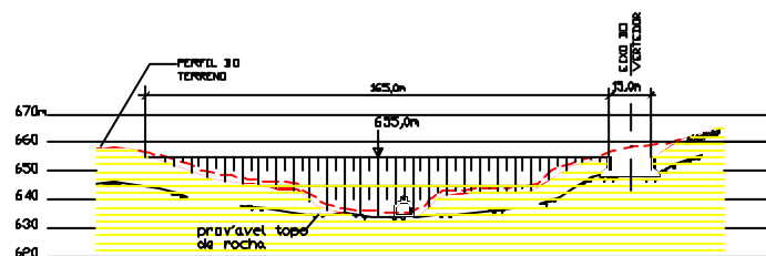
CORTE B-B ESC 1:2000
