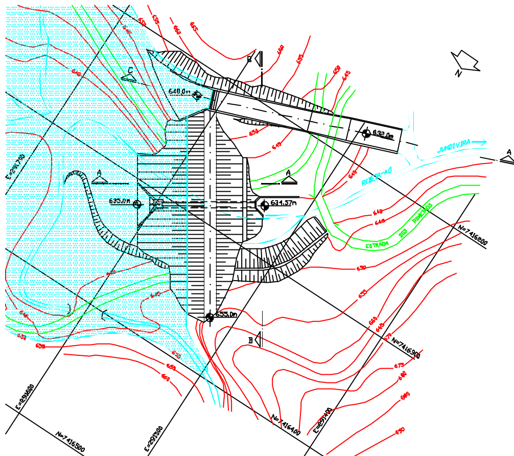
PLANTA ESC 1:2000
