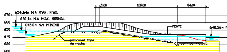
CORTE C-C ESC 1:2000
