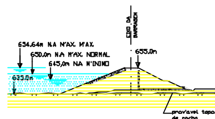
CORTE A-A ESC 1:2000
