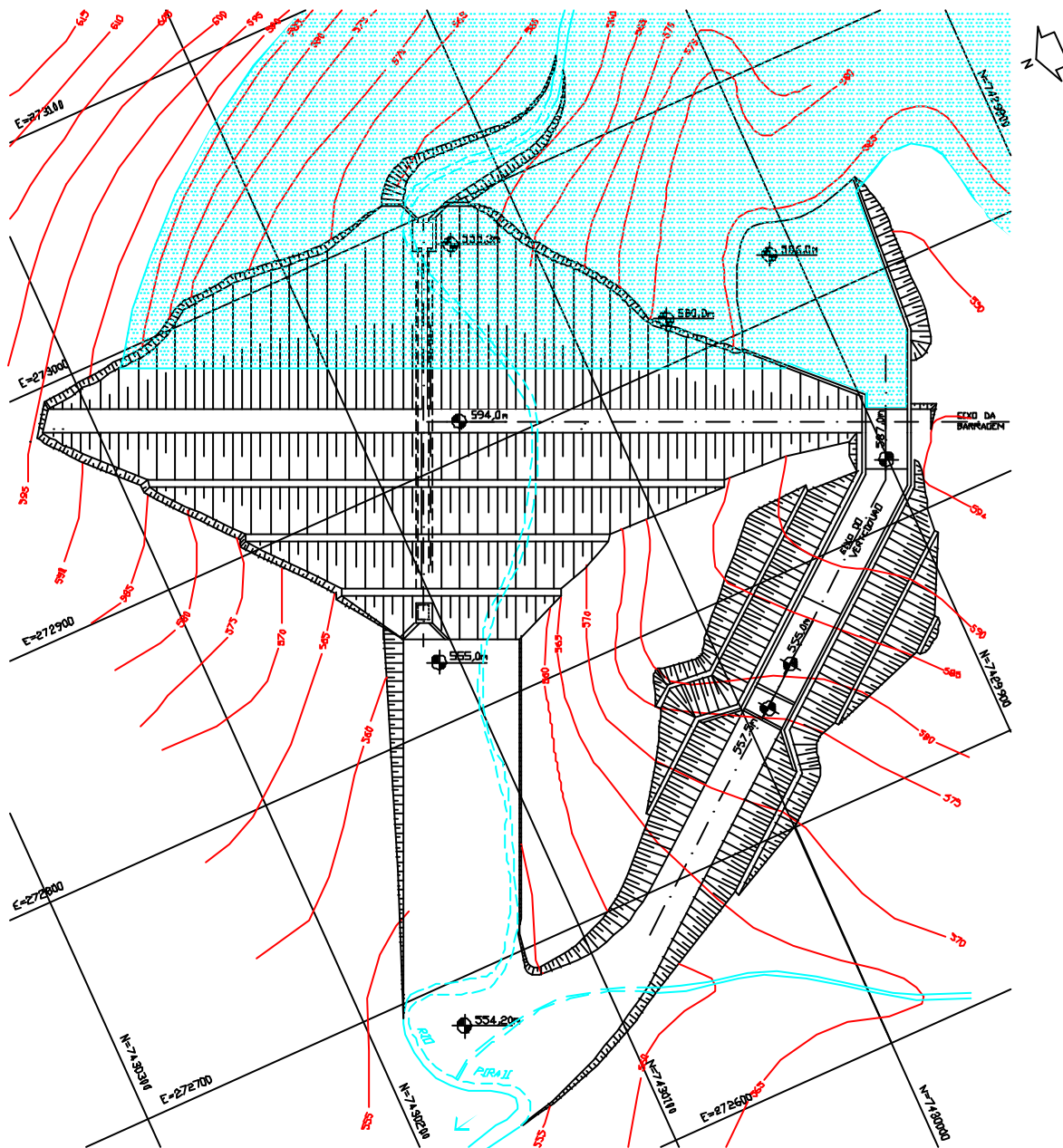
PLANTA ESC 1:2000
