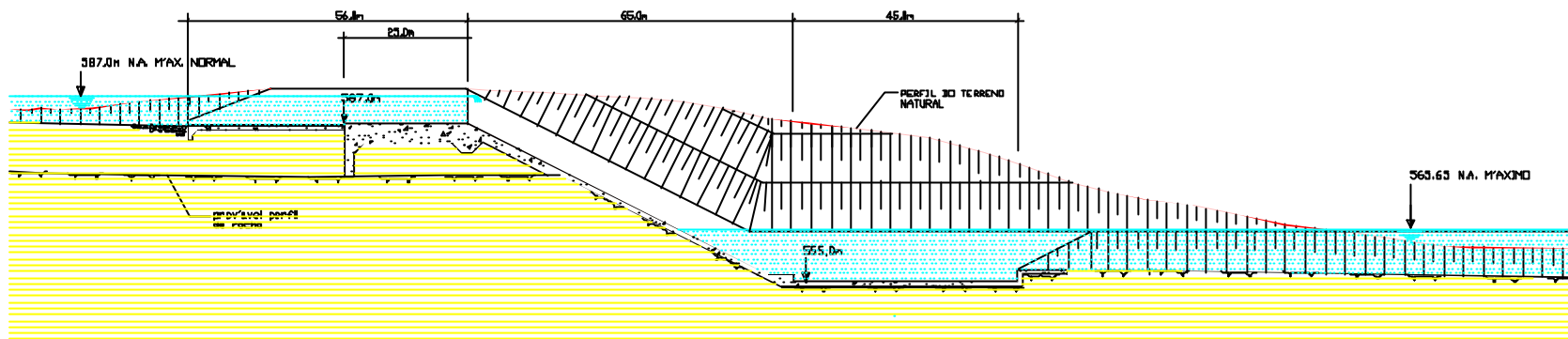
VERTEDOURO CORTE LONGITUDINAL ESC 1:1000
