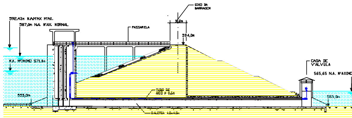
TOMADA D'ÁGUA CORTE LONGITUDINAL ESC 1:1000
