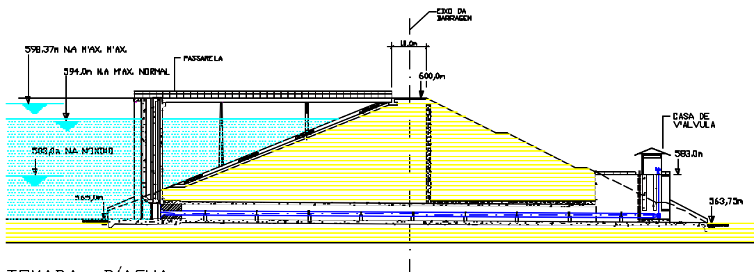
TOMADA D'ÁGUA CORTE LONGITUDINAL ESC 1:1000
