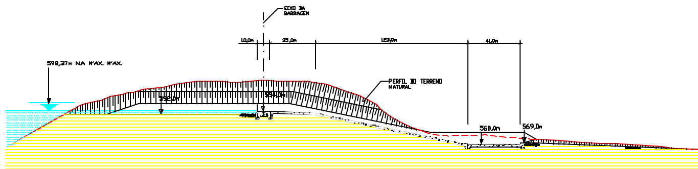
VERTEDOURO CORTE LONGITUDINAL ESC 1:2000
