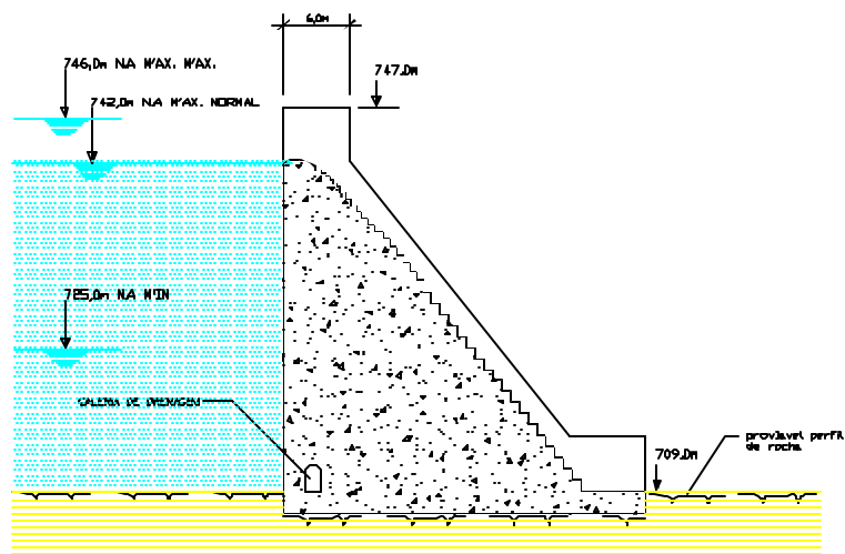
VERTEDOURO CORTE TÍPICO ESC 1:500
