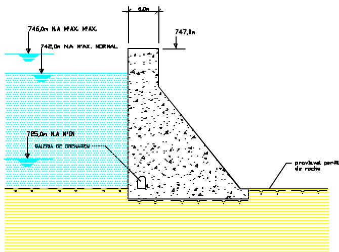
CORTE TÍPICO ESC 1:500
