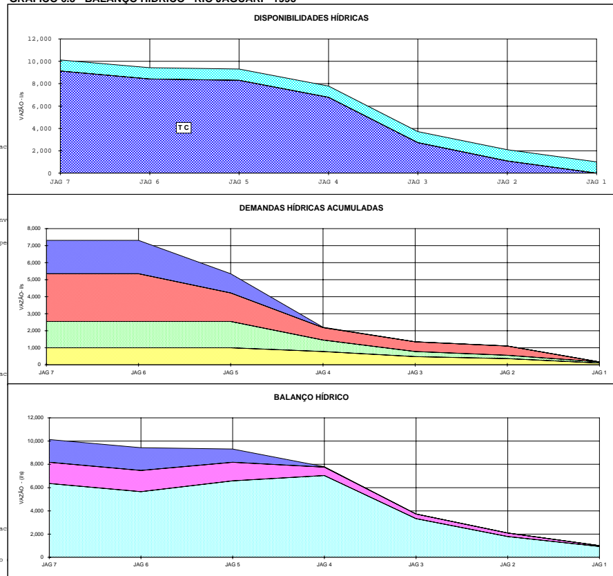
GRÁFICO 6.3 - BALANÇO HÍDRICO - RIO JAGUARI - 1995
