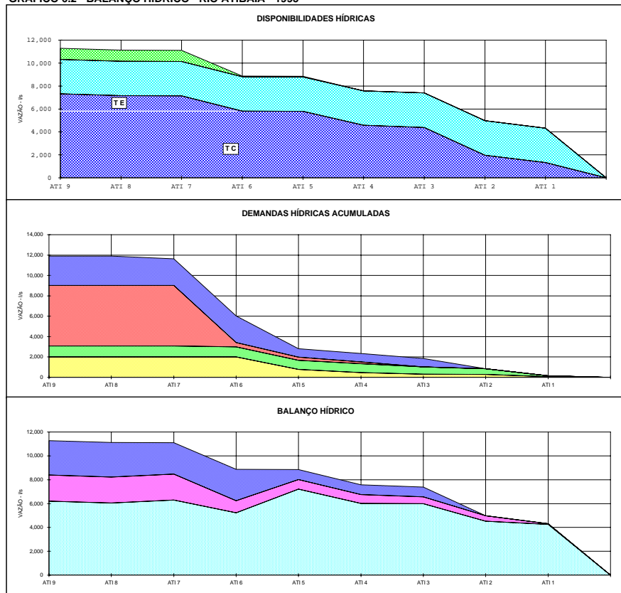
GRÁFICO 6.2 - BALANÇO HÍDRICO - RIO ATIBAIA - 1995
