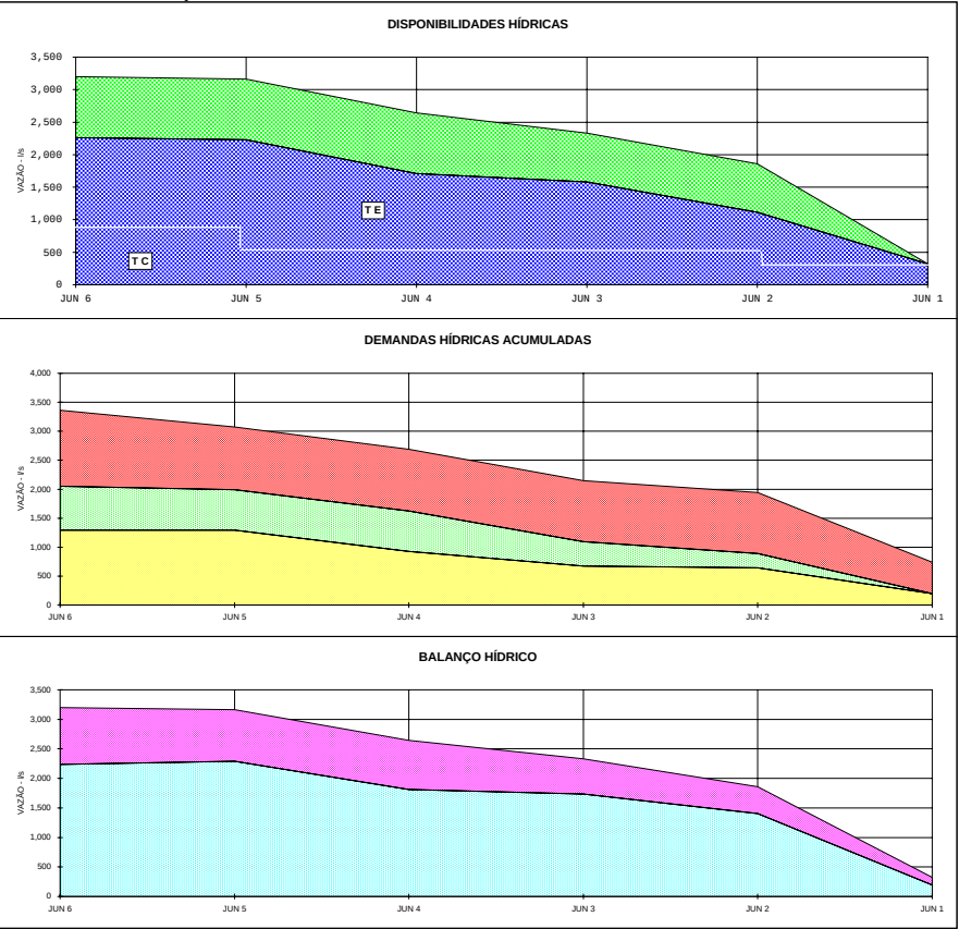
BALANÇO DE DISPONIBILIDADES X NECESSIDADES HÍDRICAS
