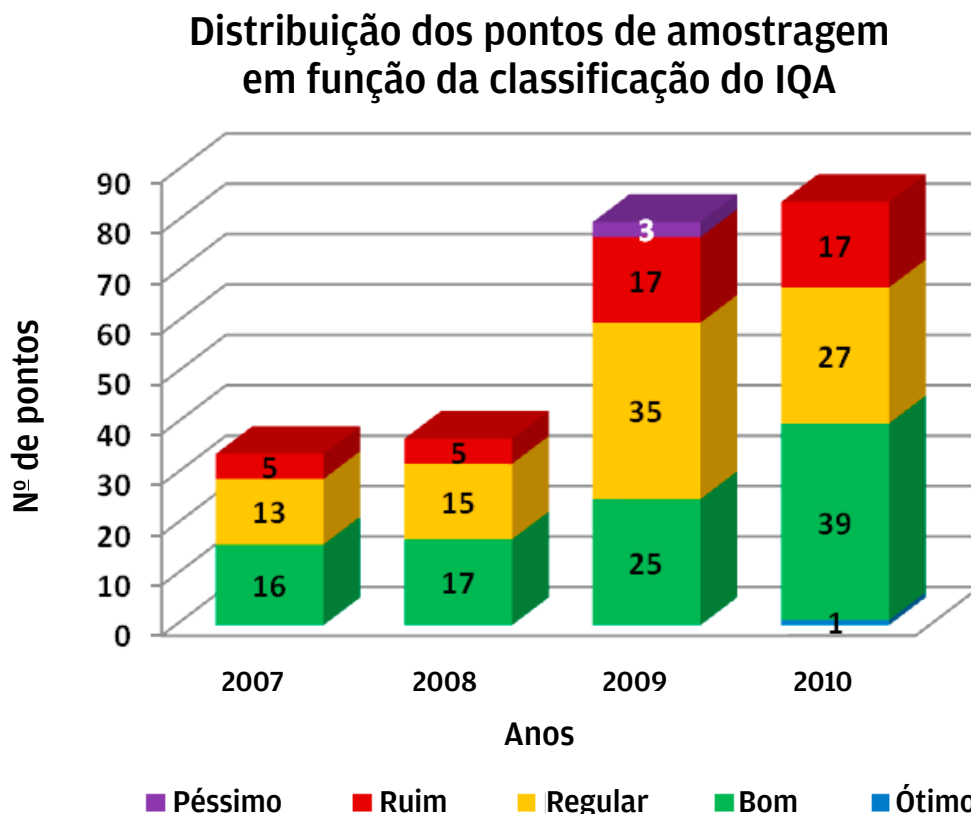
Gráfico 19: Distribuição dos pontos de amostragem em função da classificação do IQA
