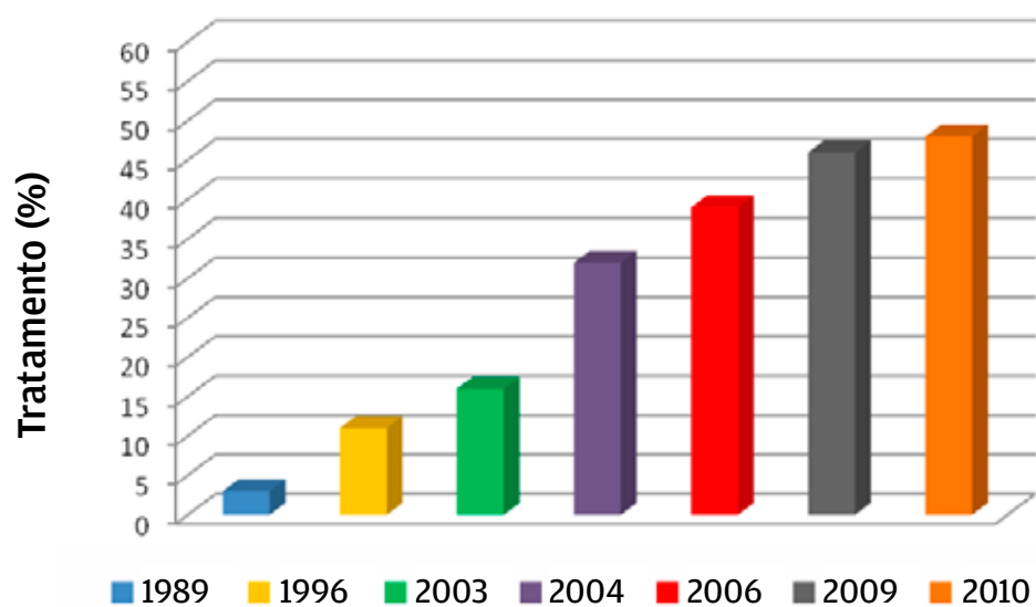
Gráfico 29: Evolução do tratamento de esgoto nas Bacias PCJ
