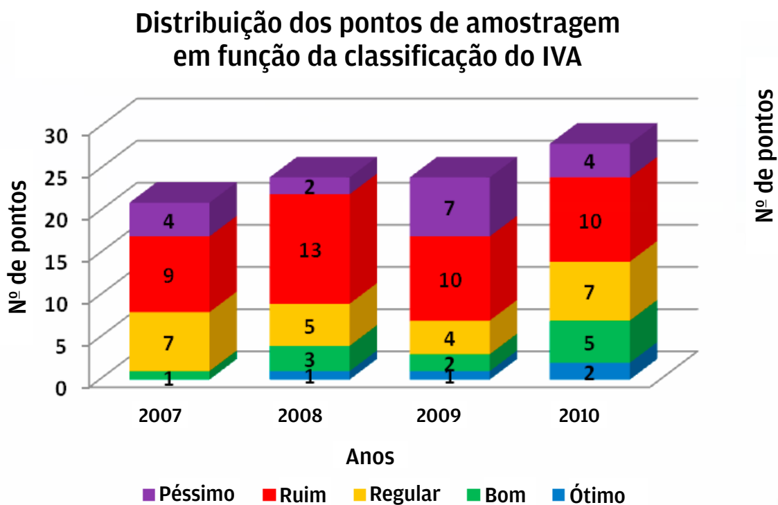
Gráfico 21: Distribuição dos pontos de amostragem em função da classificação do IVA entre 2007 e 2010
