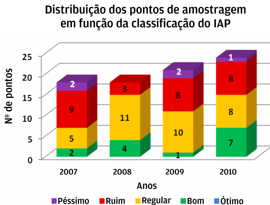
Gráfico 20: Distribuição dos pontos de amostragem em função da classificação do IAP
