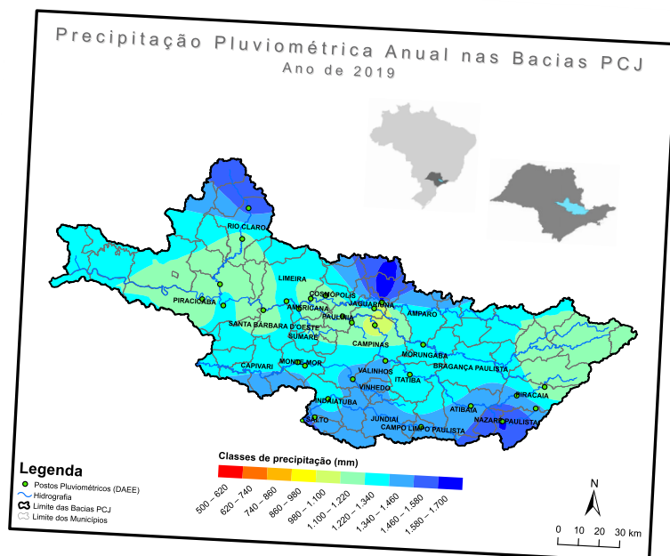
Precipitação pluviométrica anual nas Bacias PCJ
