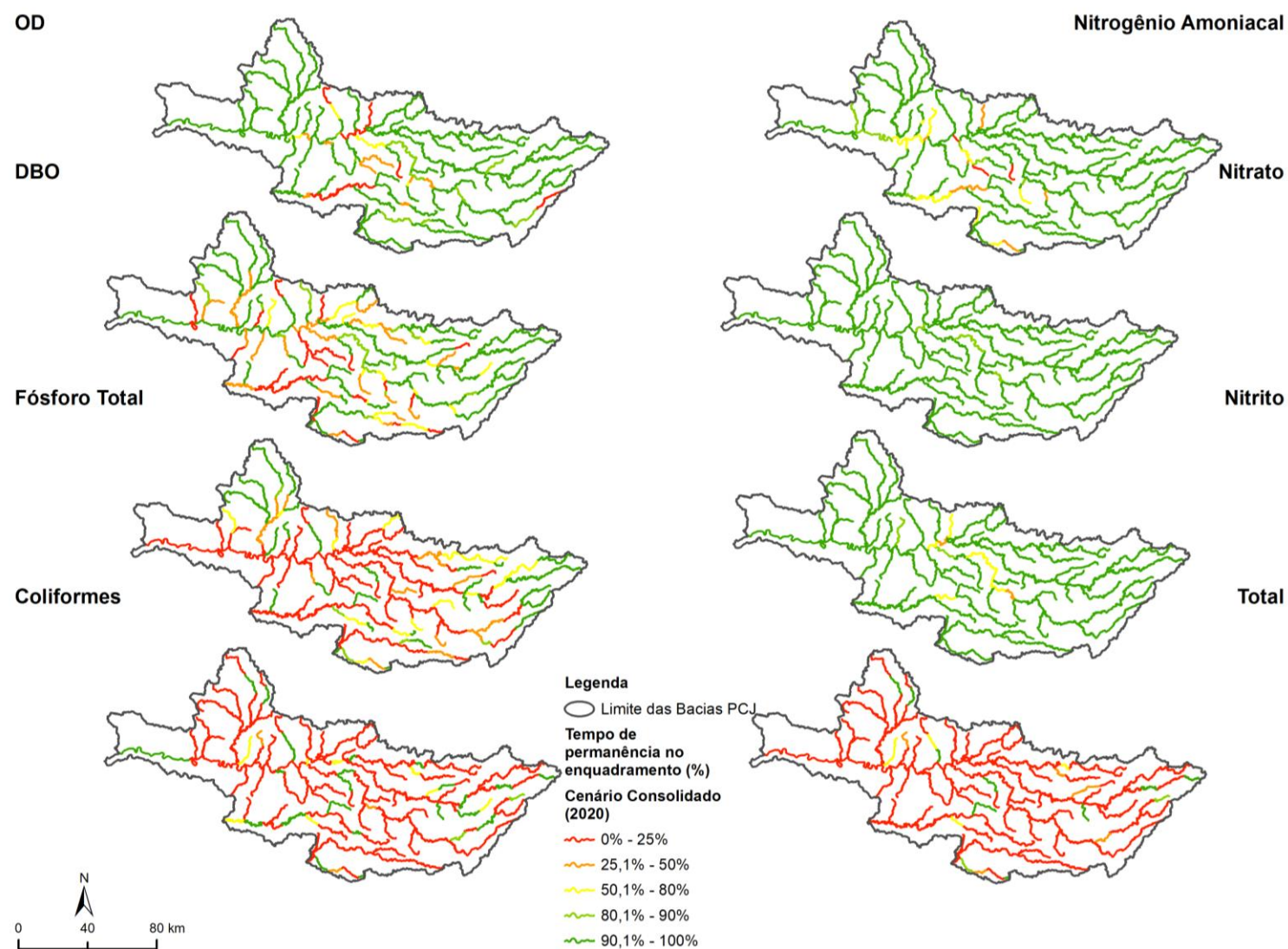
Figura 3.11 - Permanência do Enquadramento para cada parâmetro no Cenário Consolidado (2020) – Série Histórica.
