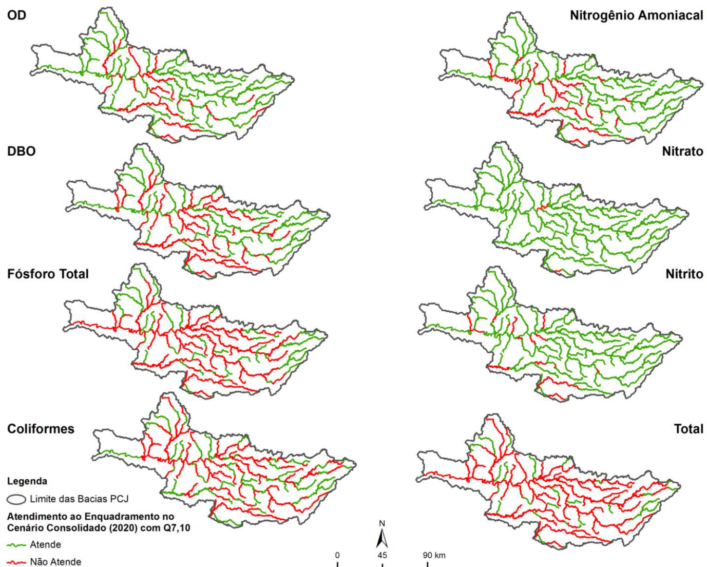
Figura 3.10 - Atendimento ao Enquadramento para cada parâmetro no Cenário Consolidado (2020) com Q_{7,10} .
