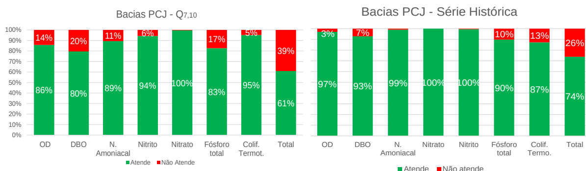
Figura 3.14 – Percentual de atendimento ao enquadramento por parâmetro nas ACs das Bacias PCJ no Cenário de Q 7,10 (2035) (esquerda) e Percentual de atendimento no tempo nas ACs das Bacias PCJ no Cenário com série histórica de vazões (direita).
