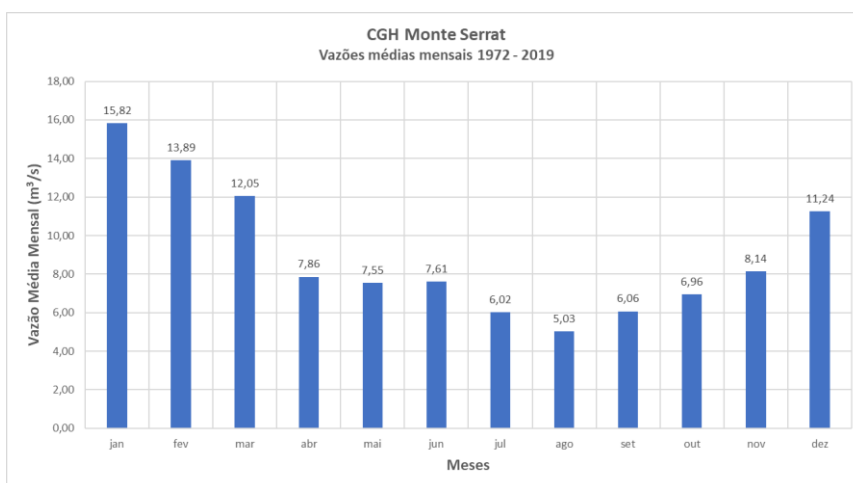
Figura 12 – Vazões Médias Mensais CGH Monte Serrat
