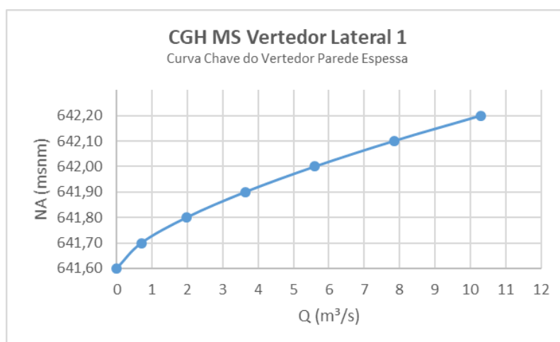
Figura 18 – Curva Chave do Vertedor Parede Espessa CGH Monte Serrat
