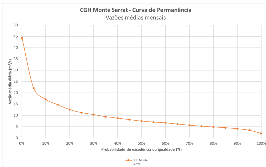
Figura 14 – Curva de Permanência CGH Monte Serrat
