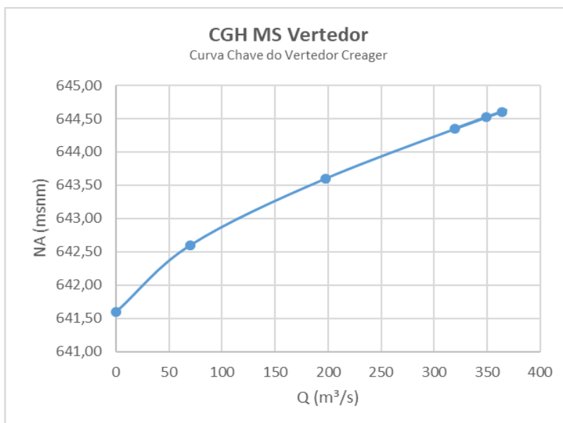
Figura 15 – Curva Chave do Vertedor Creager CGH Monte Serrat
