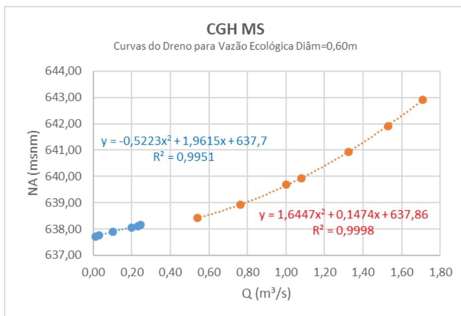
Figura 16 – Curva do Dreno Vazão Ecológica CGH Monte Serrat
