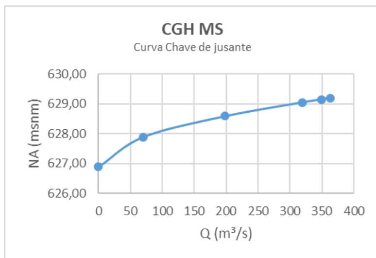
Figura 21 – Curva Chave de Jusante CGH Monte Serrat
