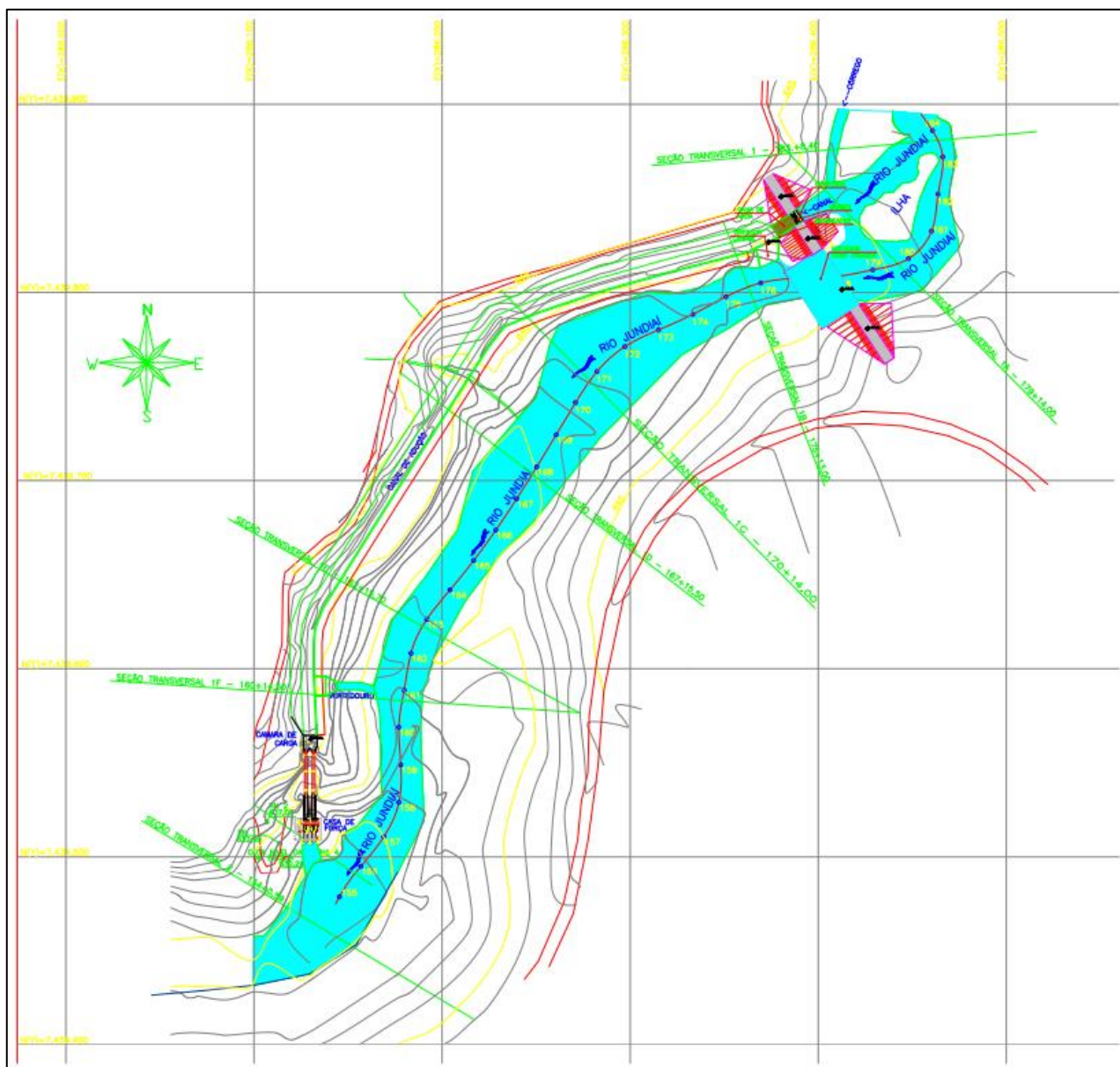
Figura 25 – Arranjo Geral do Empreendimento – CGH Monte Serrat
