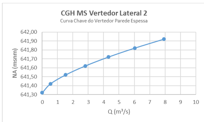
Figura 20 – Curva Chave do Vertedor Parede Espessa CGH Monte Serrat
