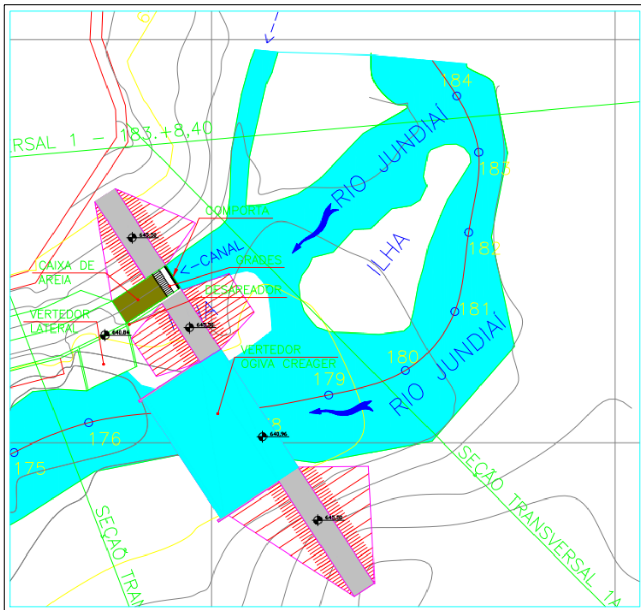
Figura 27 – Barramento Planta – CGH Monte Serrat
