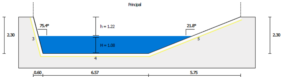
Figura 19 – Canal de Adução CGH Monte Serrat
