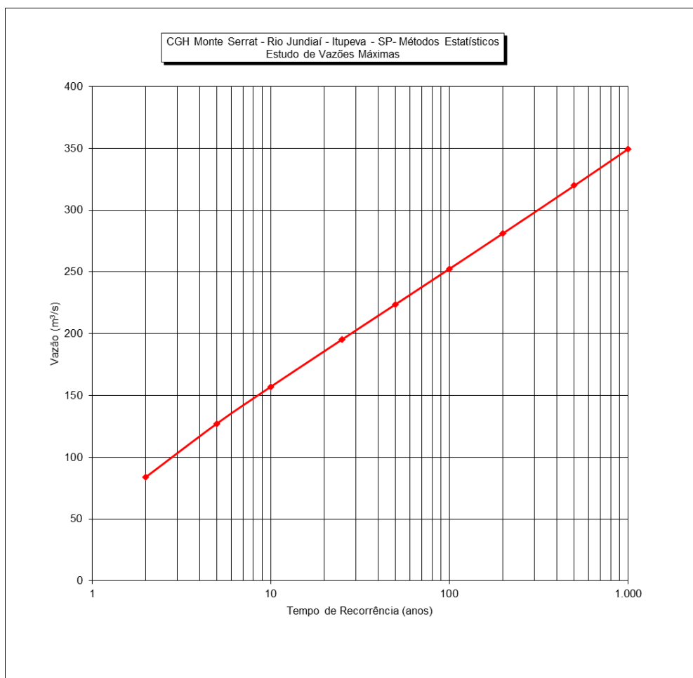
Figura 13 – Estudos Estatísticos CGH Monte Serrat
