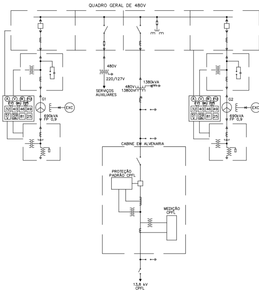
Figura 24 – Diagrama Simplificado Conexão – Rede Interna CGH Monte Serrat
