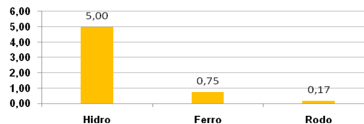
Modais de transporte: Eficiência energética – Carga / Potência (t / hp)
